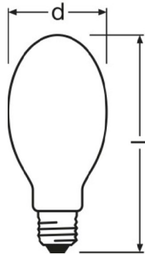
NAV E/I 70 W/I E27, NAV E 150 W E40, NAV E 250 W E40, NAV E 400 W E40
